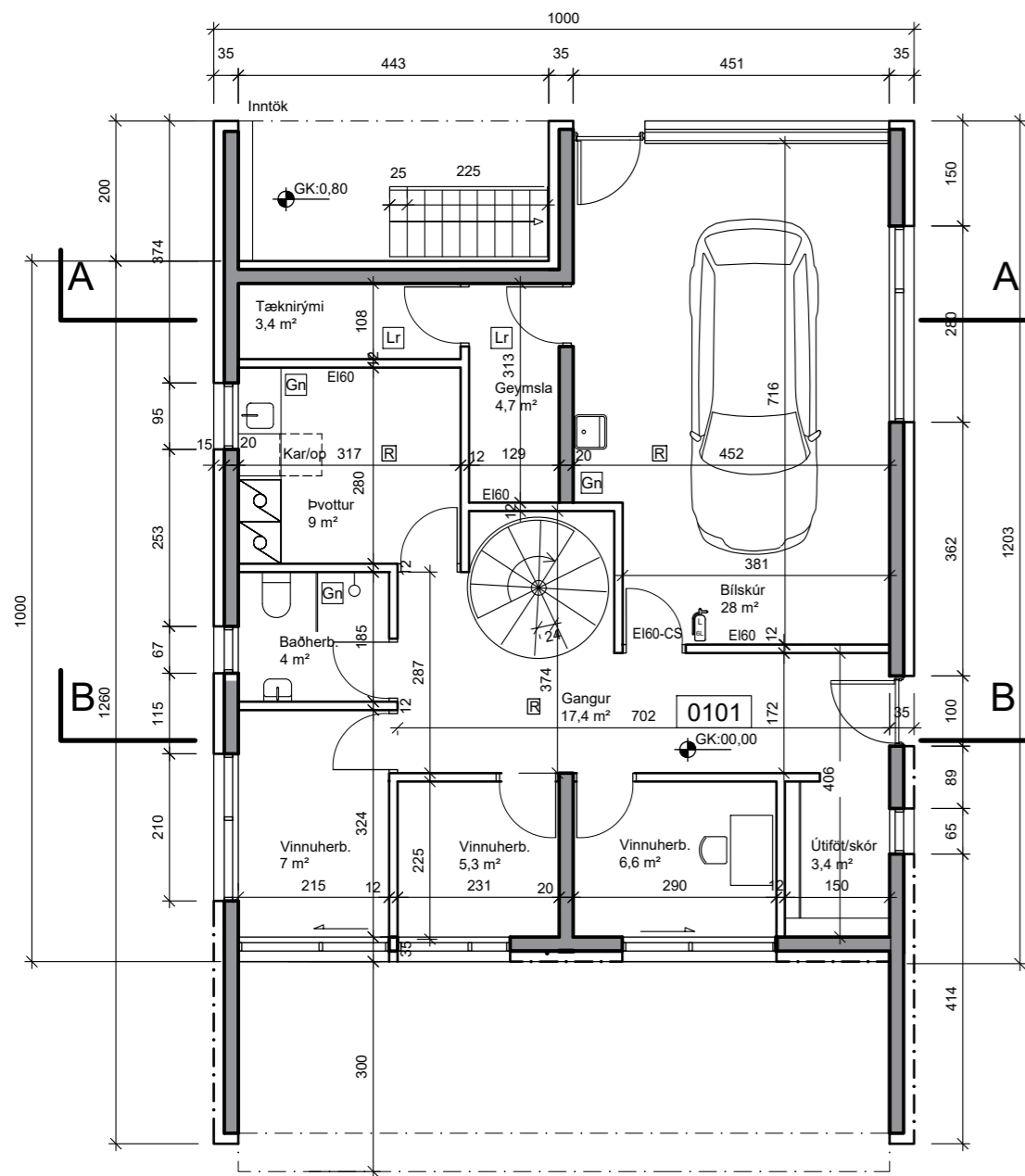
Grunnmynd 1.hæðar 1:100
