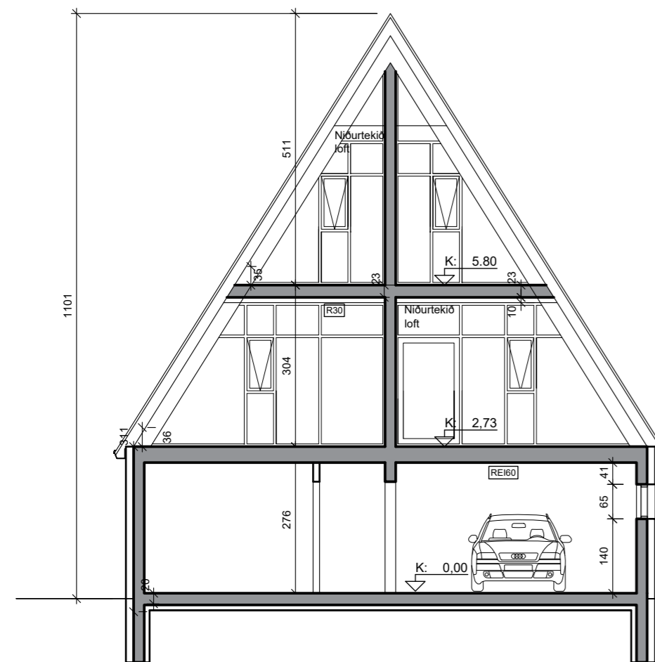
Sneiðing A-A 1:100
