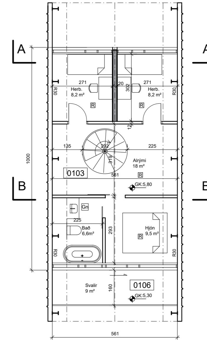
Grunnmynd 3.hæðar 1:100
