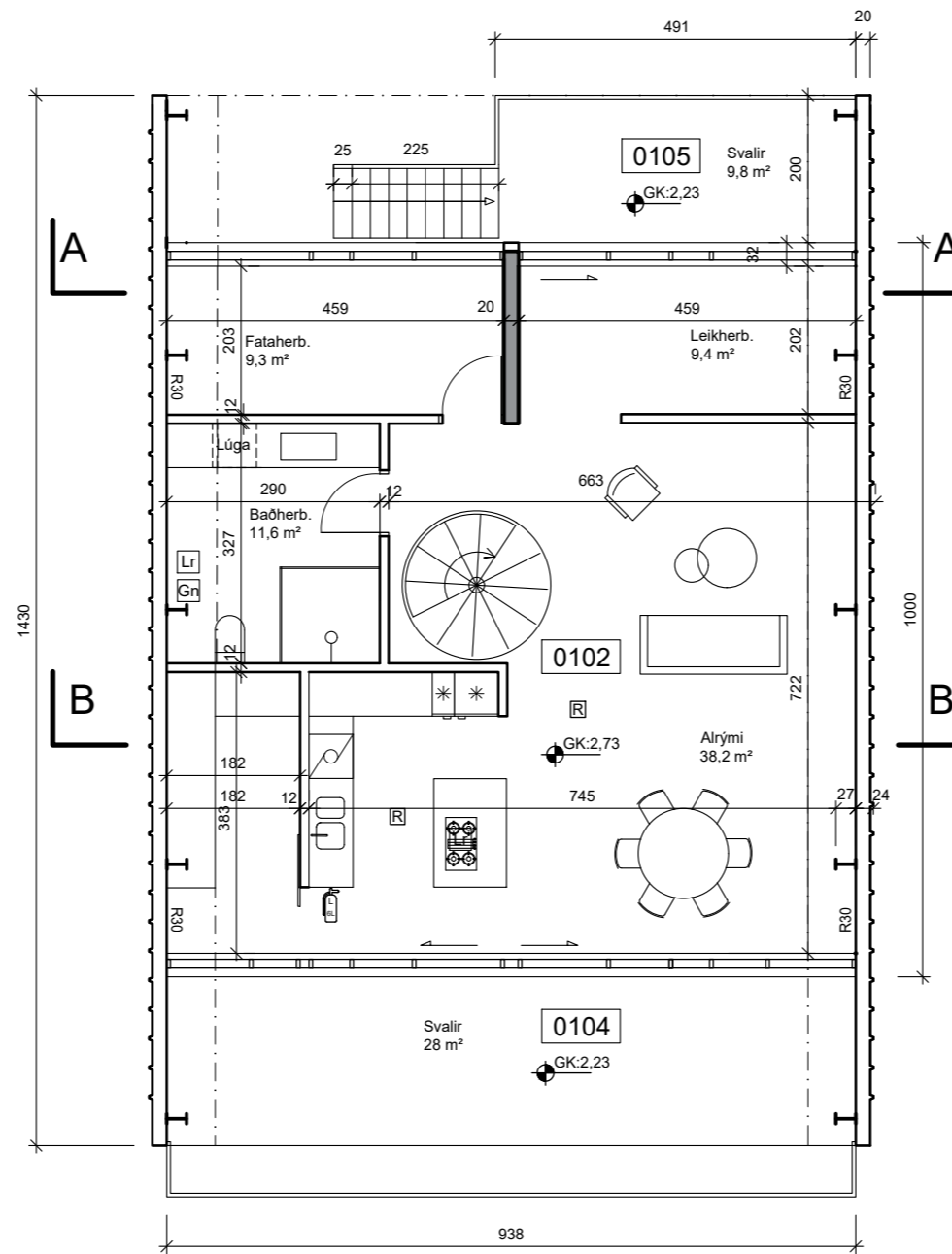
Grunnmynd 2.hæðar 1:100
