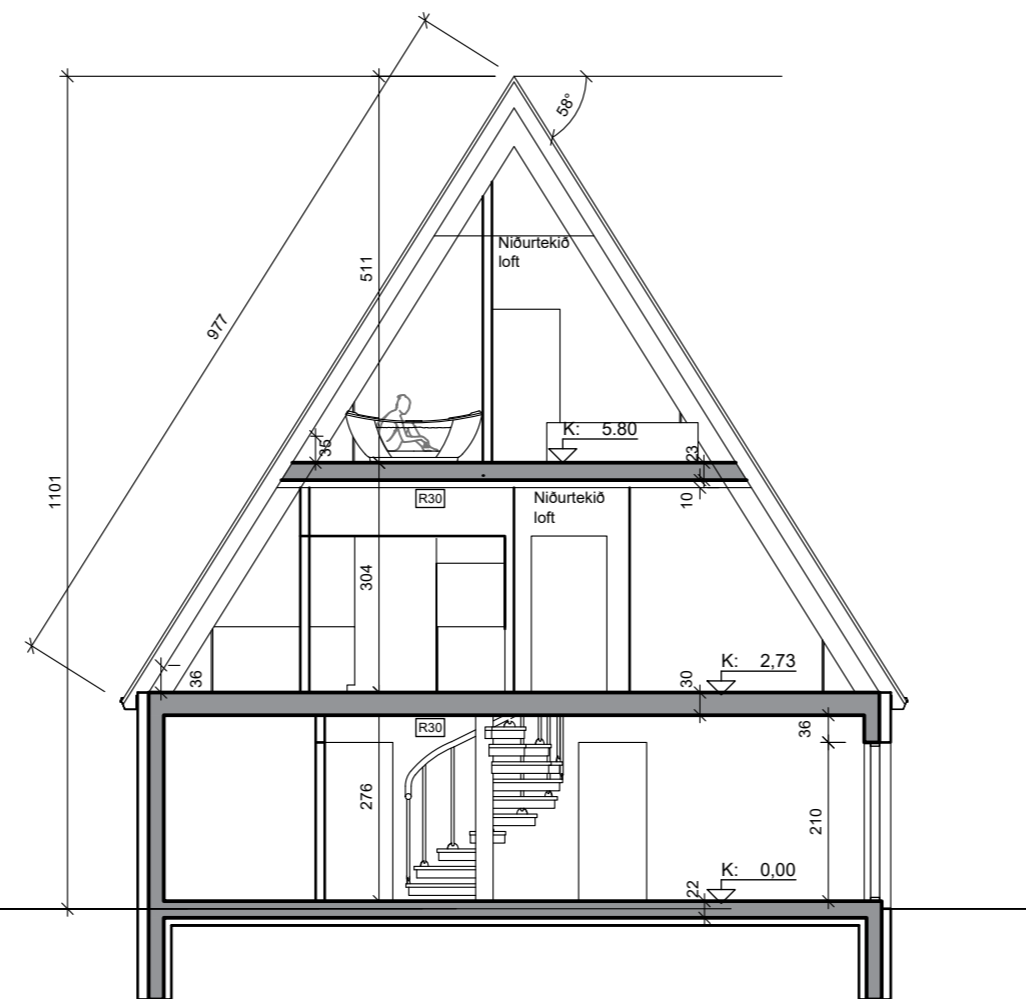
Sneiðing B-B 1:100
