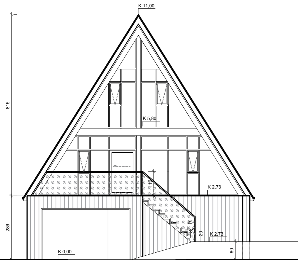
Úlit-Norður 1:100
