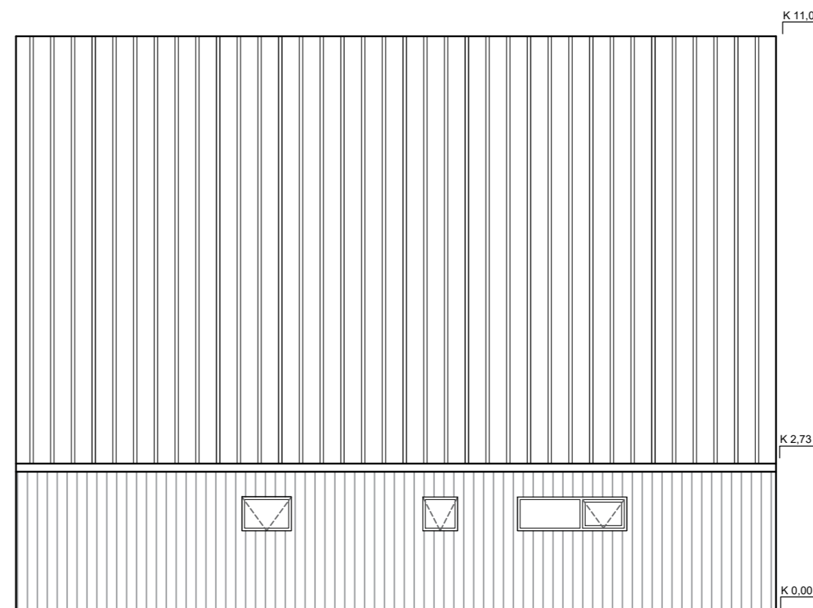
Úlit-Austur 1:100
