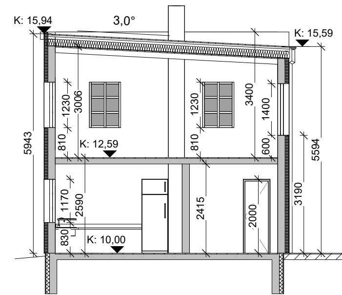
Snið A 1 : 100
