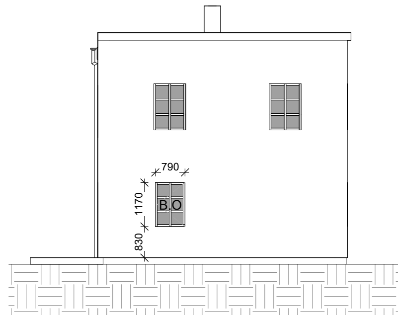
Vestur 1 : 100
