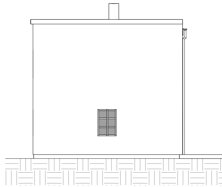
Austur 1 : 100
