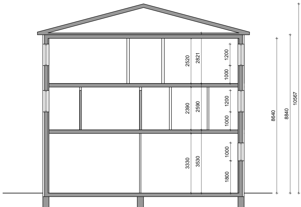
Snið A-A 1 : 100
